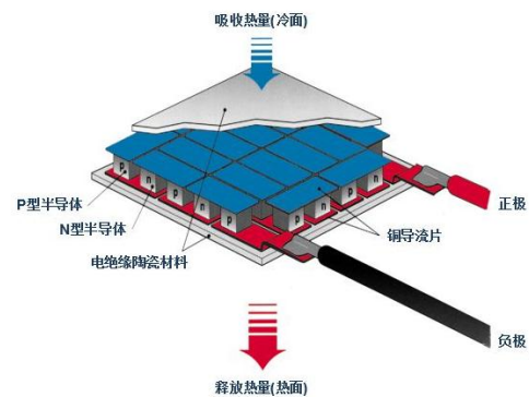
制冷片原理图
